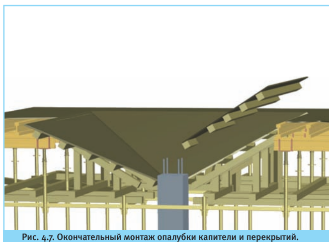
Рис. 4.7. Окончательный монтаж опалубки капители и перекрытий.
