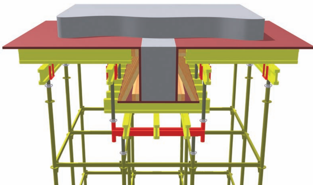
Рис. 3.6 Монтаж формообразующих элементов балки и плиты
