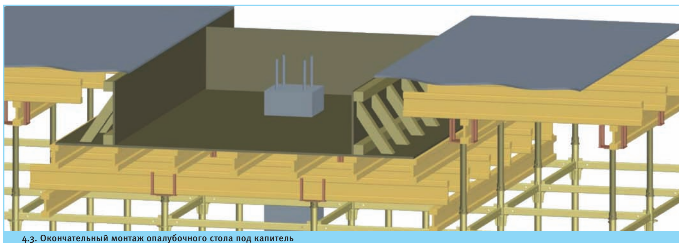
4.3. Окончательный монтаж опалубочного стола под капитель
