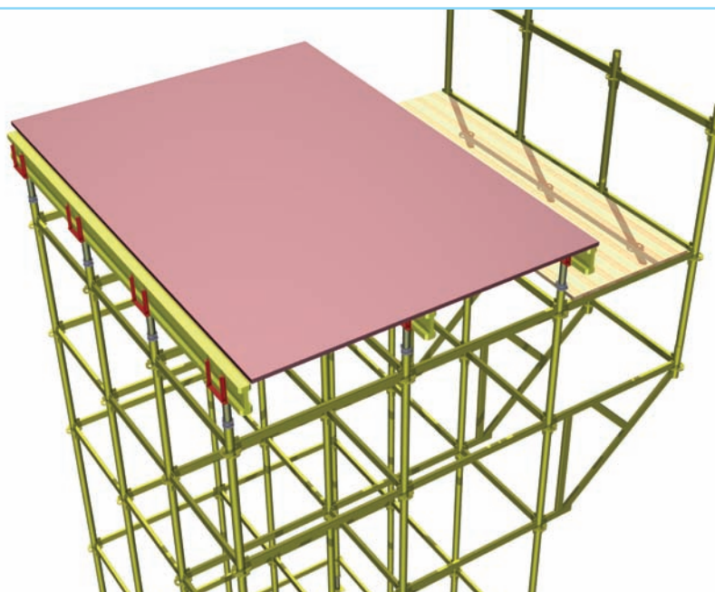
Рис. 3.4 Монтаж опалубки под разновеликие ж.б. балки.
