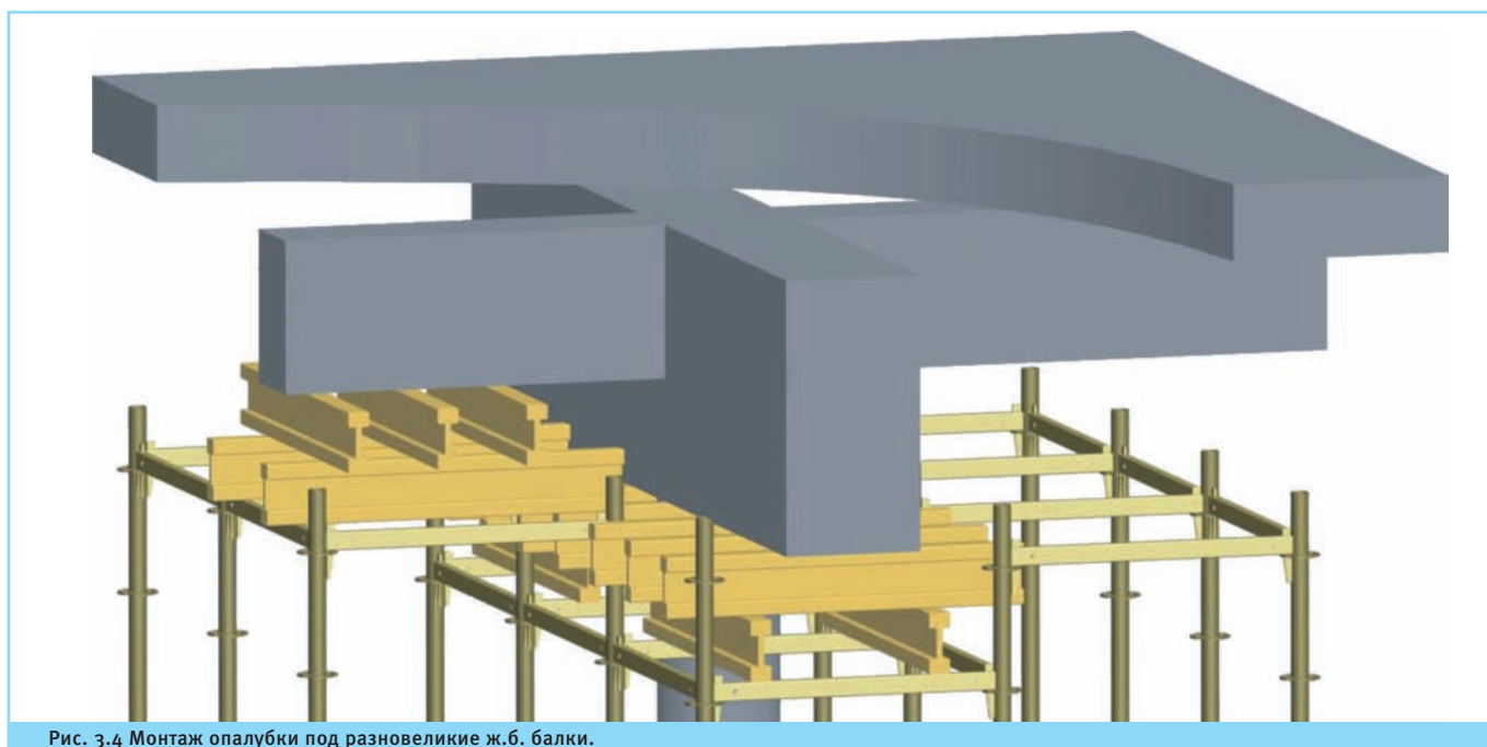
Рис. 3.4 Монтаж опалубки под разновеликие ж.б. балки.
