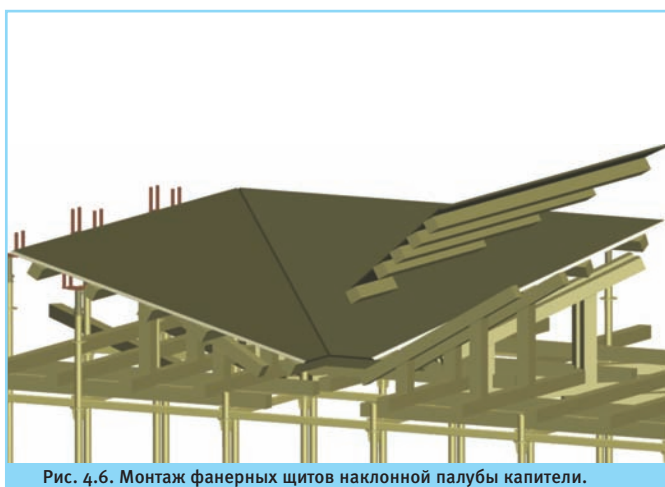
Рис. 4.6. Монтаж фанерных щитов наклонной палубы капители.
