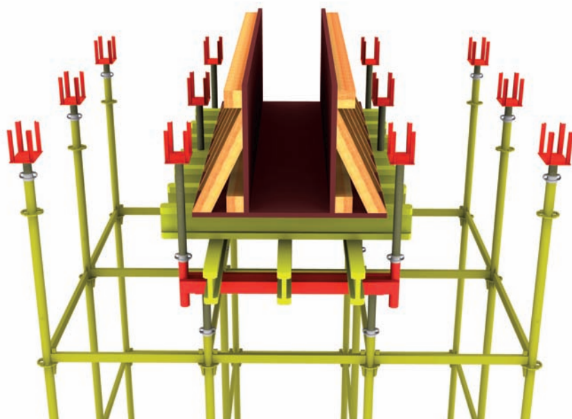
Рис. 3.5 Монтаж формообразующих элементов балки
