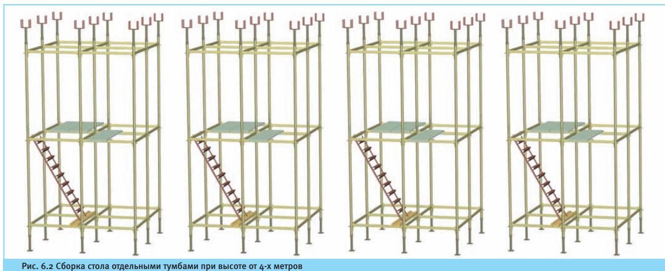
Рис. 6.2 Сборка стола отдельными тумбами при высоте от 4-х метров
