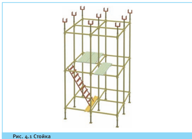
Рис. 4.1 Стойка
