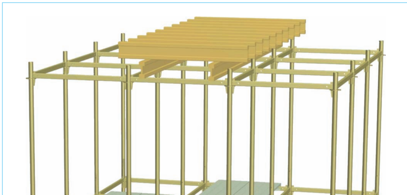
Рис. 3.1 Продольный и поперечный набор опалубки ж.б. балки.
