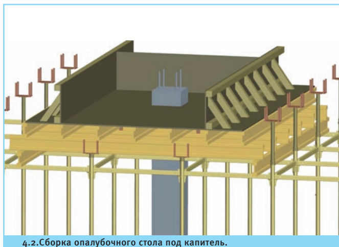
4.2. Сборка опалубочного стола под капитель.
