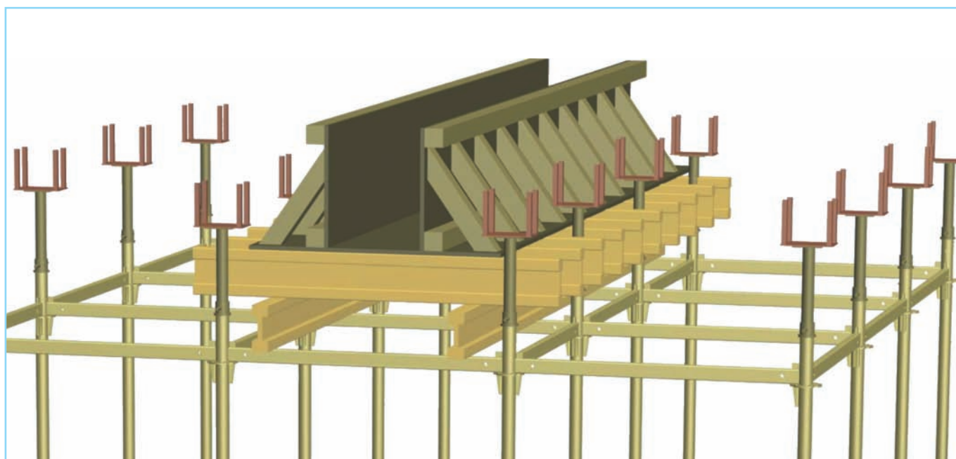
Рис. 3.2 Монтаж фанеры.
