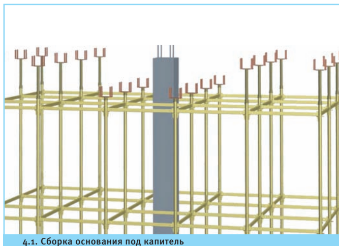
4.1. Сборка основания под капитель
