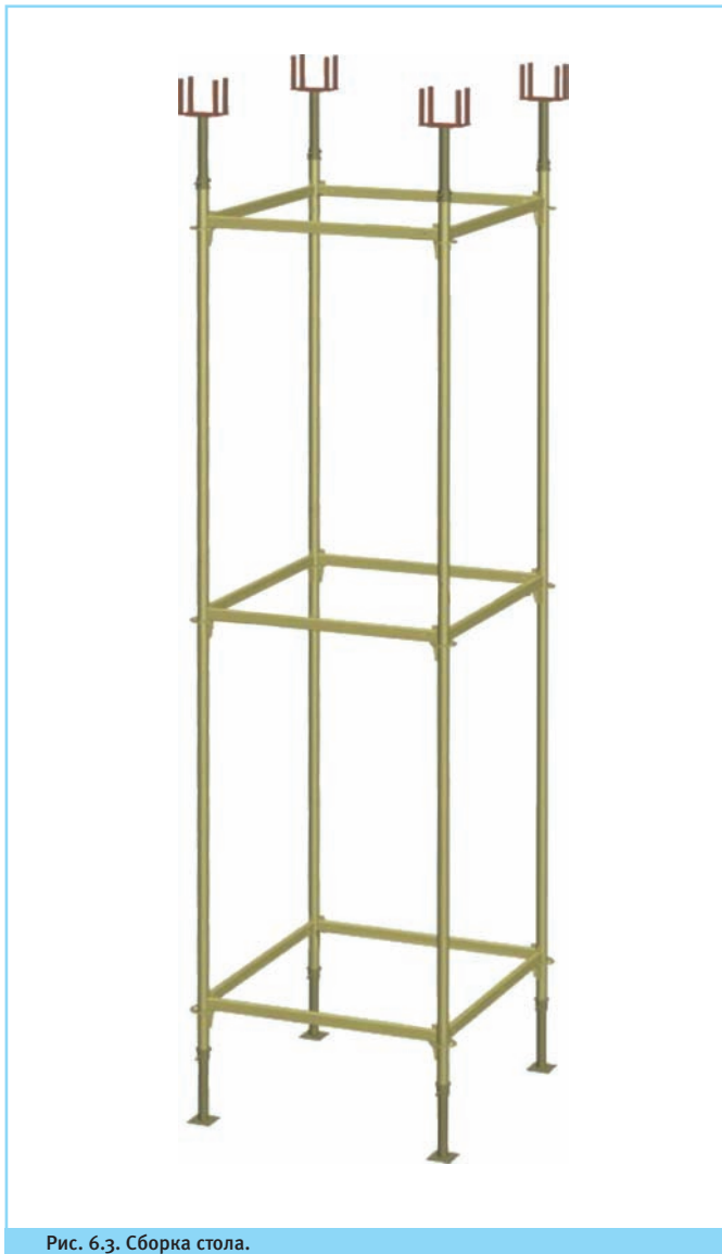
Рис. 6.3. Сборка стола.
